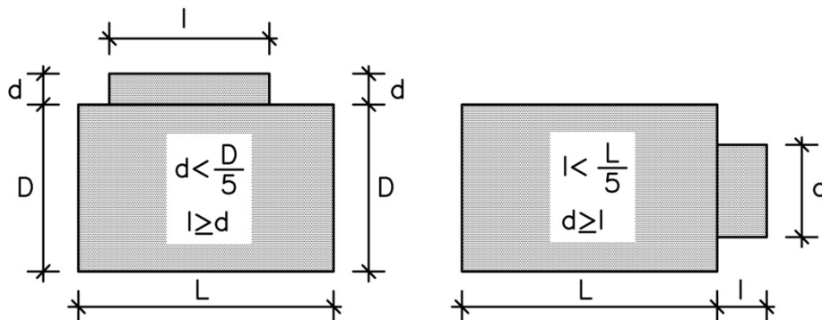
الف) پیش‌آمدگی در امتداد طول ساختمان (ب) پیش‌آمدگی در امتداد عرض ساختمان شکل ۷-۱ ابعاد پیش‌آمدگی در پلان ساختمان
